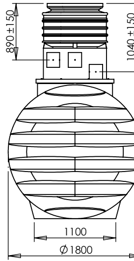
zbiornik 6000l / 6000l tank
