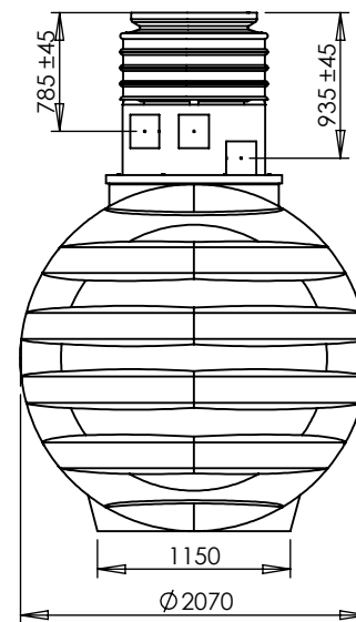
zbiornik 6000l / 6000l tank
