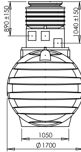
zbiornik 4500l / 4500l tank
