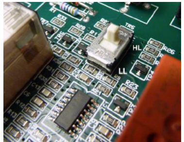
Placering av failsafe brytare på kretskortet.
