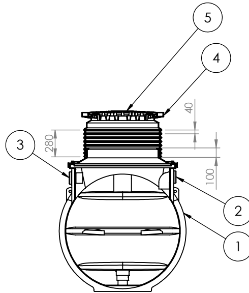
PRZEKRÓJ / SECTION A-A
